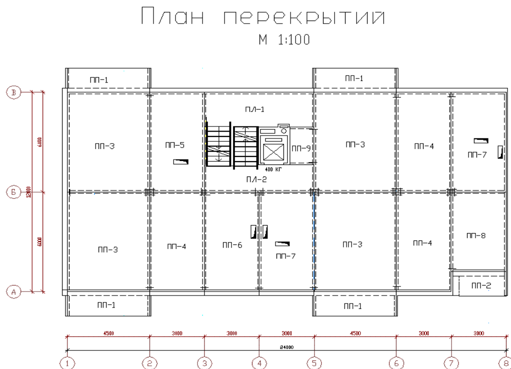
Рисунок 7 – План перекрытия бескаркасного крупнопанельного здания
