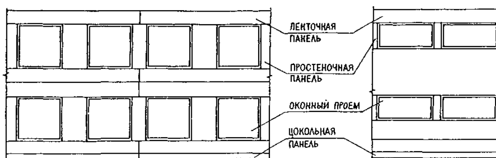
Рисунок 6 – Двухрядная разрезка
