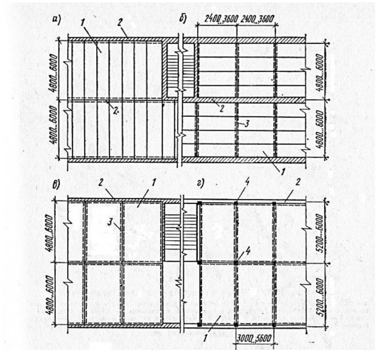
Рисунок 1 – Конструктивные схемы бескаркасных зданий
