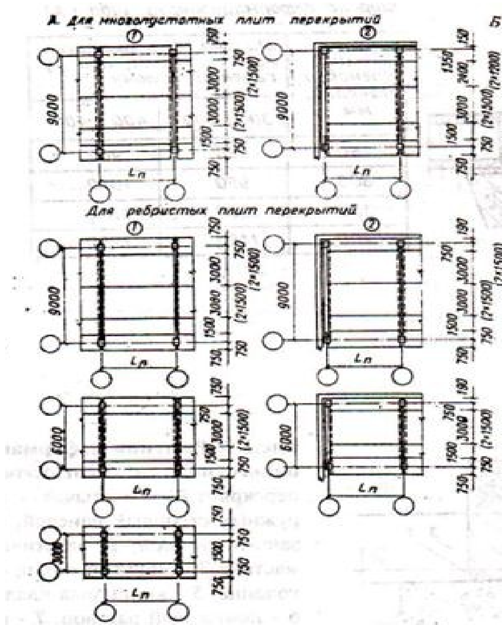
Рисунок 7 – Примеры решений планов перекрытий
