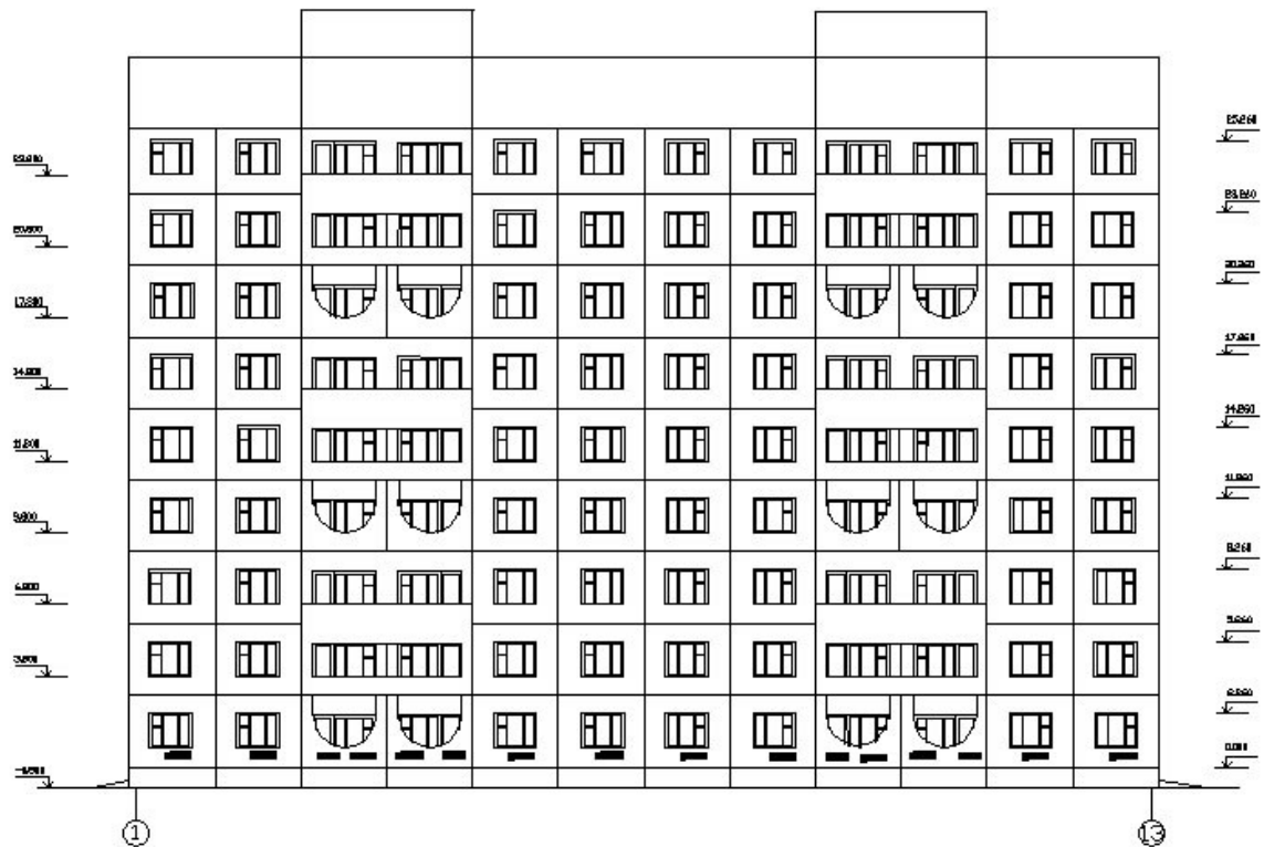
Фасад в осях 1-13
