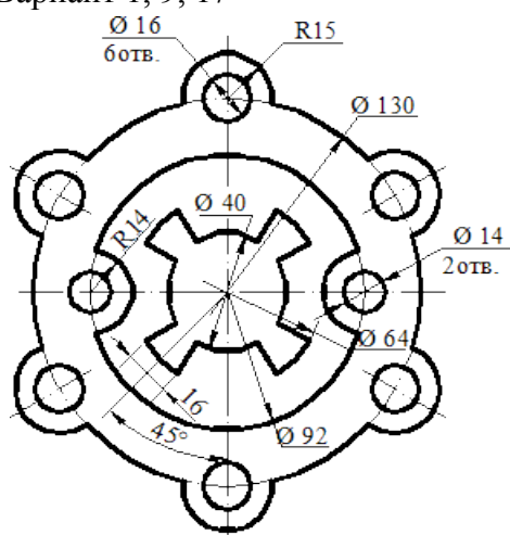
Крышка
