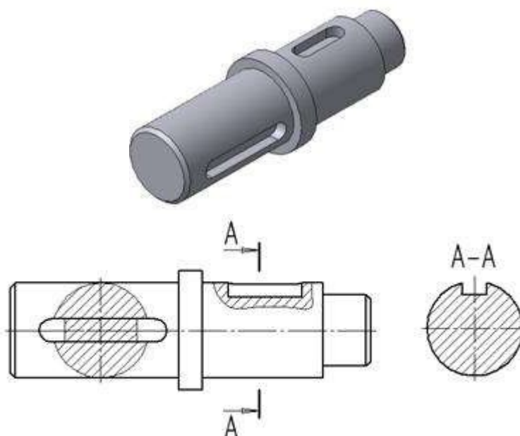
Рис.119 Построение сечений
