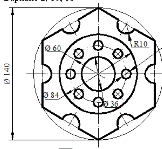
Пластина
