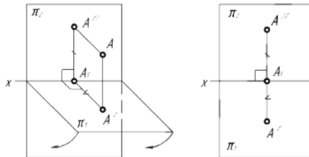
Рисунок 4.1 – Образование чертежа в системе плоскостей проекций \pi_1, \pi_2
