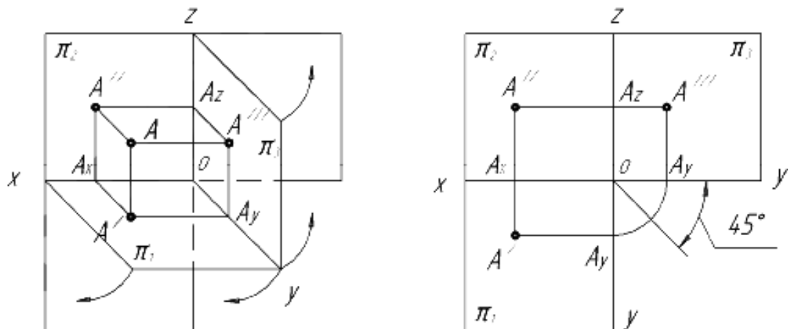
Рисунок 4.2 – Образование комплексного чертежа в системе плоскостей проекций \pi_1, \pi_2, \pi_3
