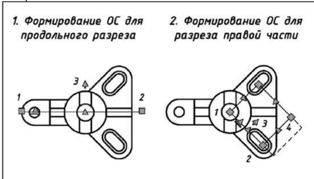
Рис. 2.33. Шаги формирования сложного ломаного разреза детали командой SECTIONPLANE (СЕКПЛОСКОСТЬ)
