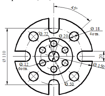
Фланец
