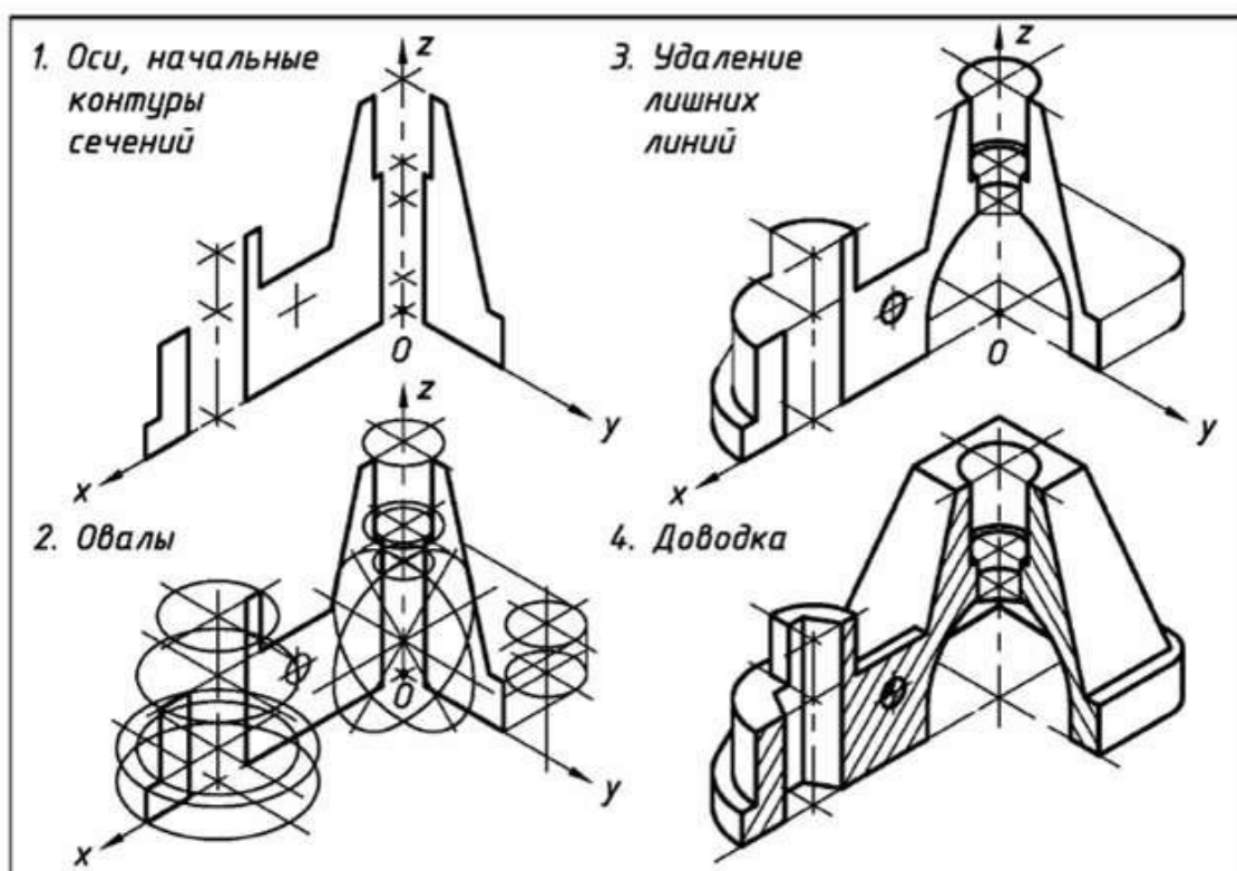
Рис. 1.35. Этапы построения чертежа детали в изометрии прямоугольной с вырезами плоскостями xoz и uoy (вариант исходных условий - рис. 1.27)
