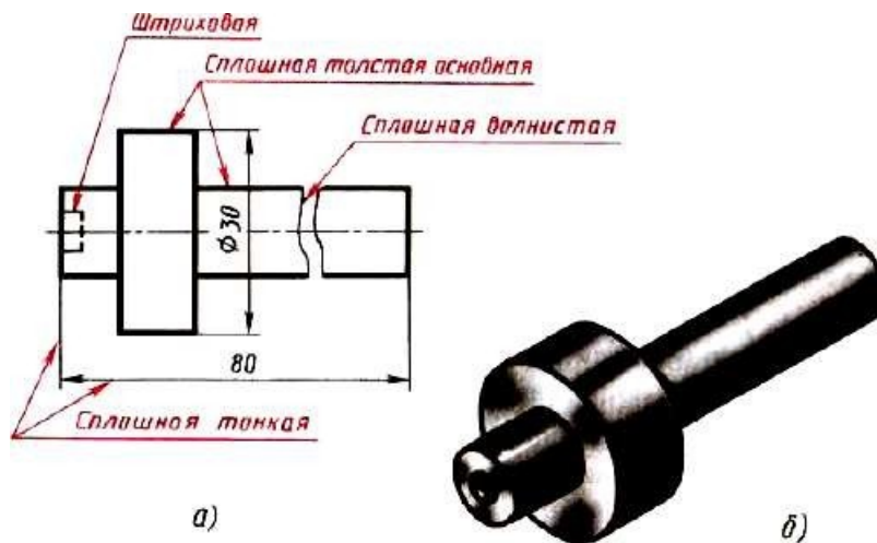
Рисунок 2.5 - Линии чертежа
