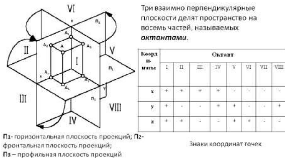
Рисунок 4.6 – Пространственная модель координатных плоскостей проекций
