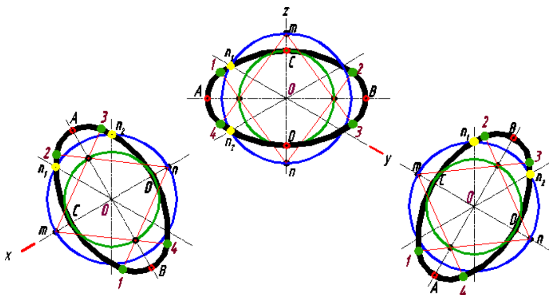
Рисунок 10.6 – Проецирование цилиндра
