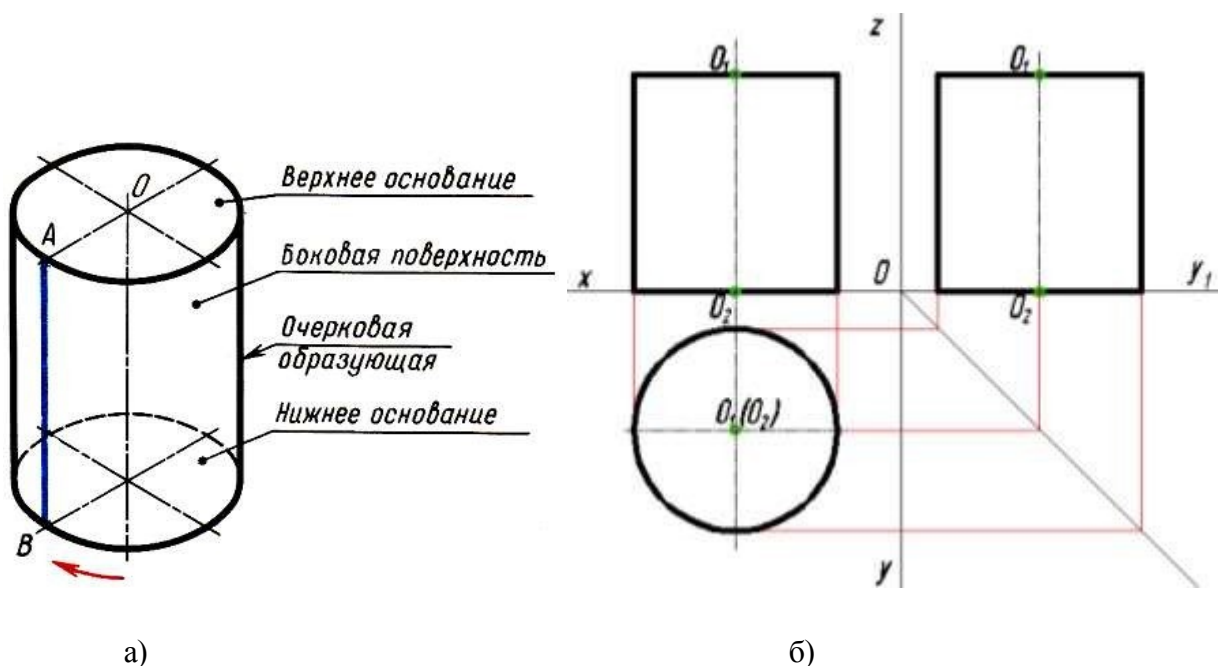
Рисунок 10.1 – Проецирование цилиндра
