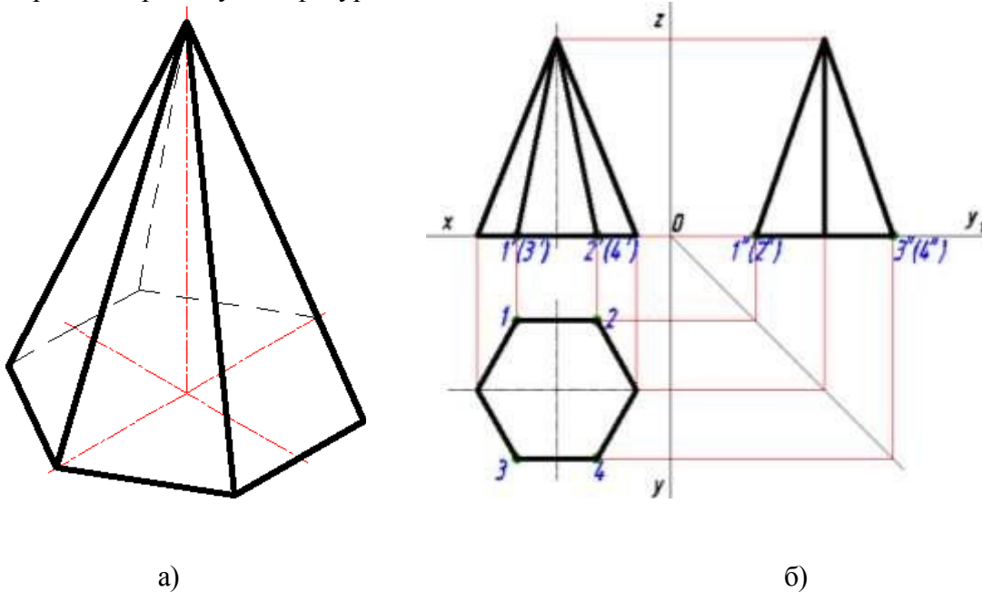
Рисунок 10.3 – Проецирование пирамиды
