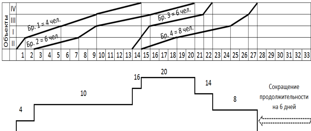
Рисунок 3—Циклограмма неритмичного потока и график потребности рабочих
