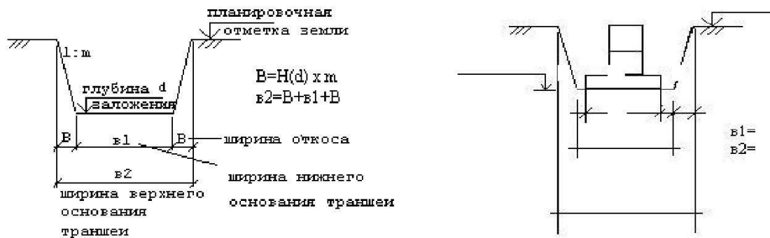
Рисунок 2 – Определение объема траншей
