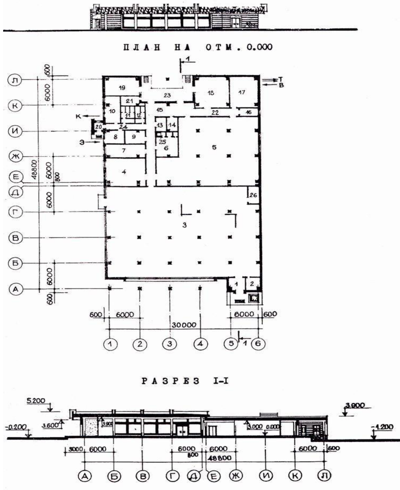
Рисунок 3—Схема здания
