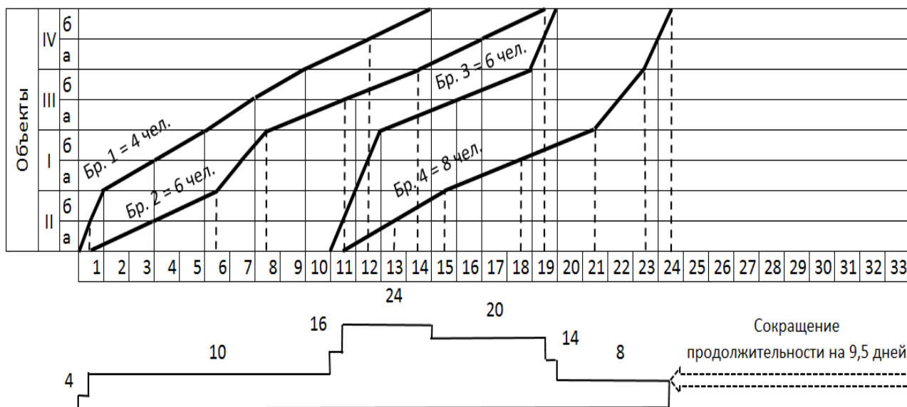
Рисунок 5— Циклограмма неритмичного потока и график потребности рабочих
