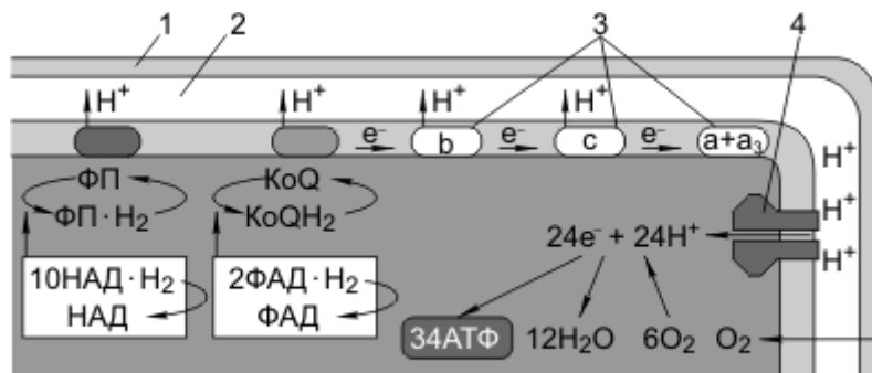
12H 2 + 6O 2 → Дыхательная цепь → 12H 2 O + 34АТФ + Q T 1 — наружная мембрана; 2 — межмембранное пространство, протонный резервуар; 3 — цитохромы; 4 — АТФ-синтетаза.
