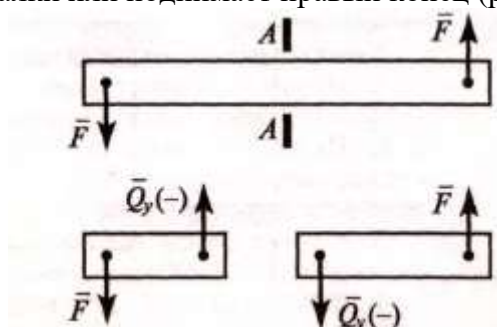
Рисунок 2 –Правила знаков для отрицательных поперечных сил
