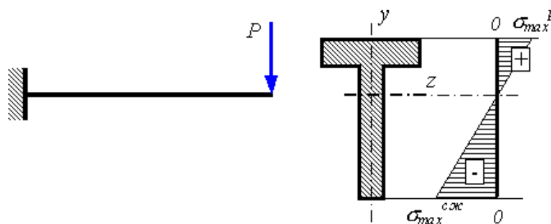
Рисунок 7 – Напряженное состояние в тавровой балке
