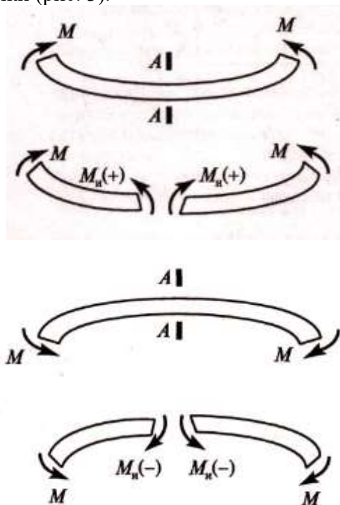
Рисунок 3 –Правила знаков для изгибающих моментов
