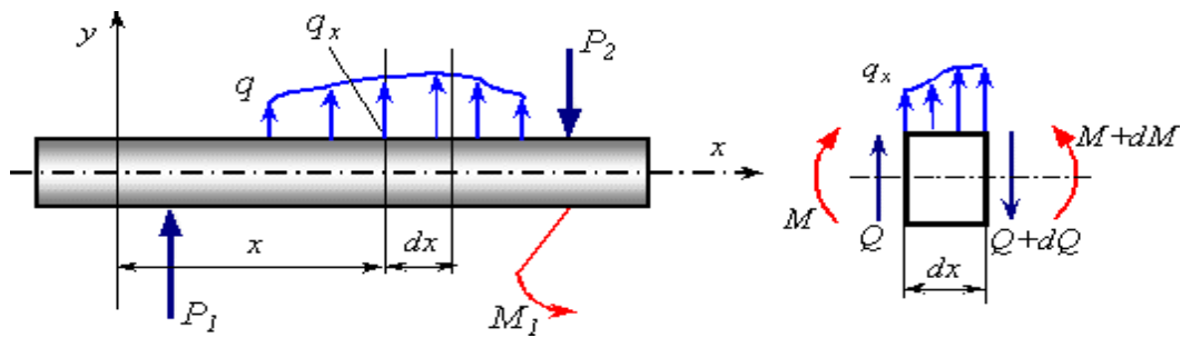
Рис. 5 – Плоский прямой изгиб
