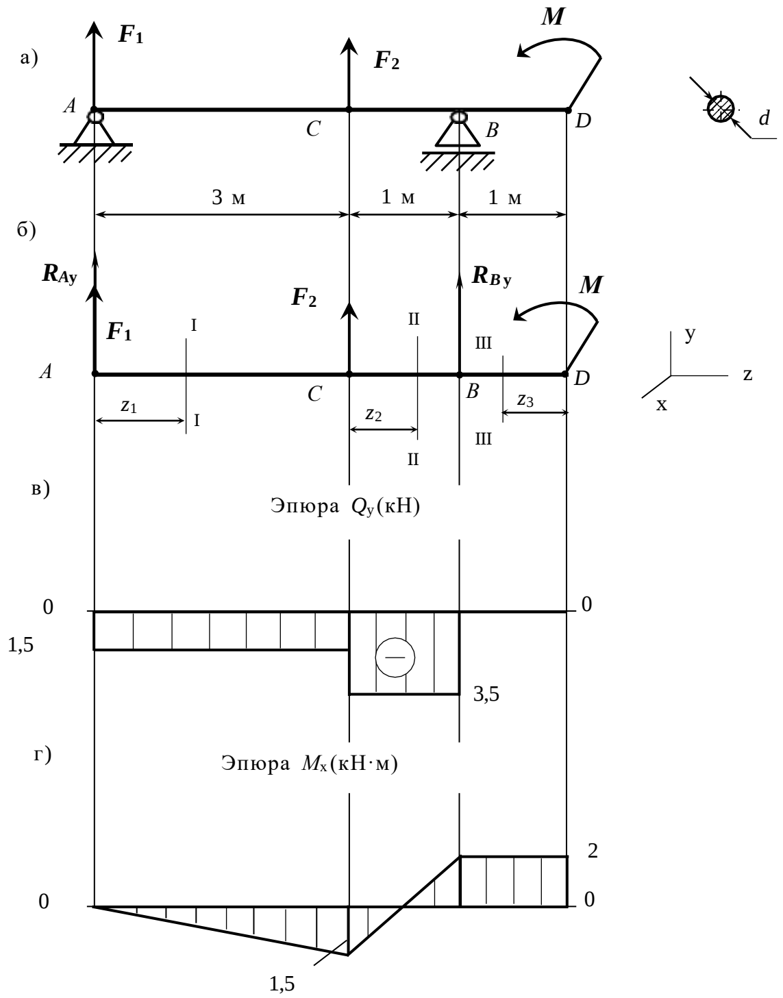
Рис. 2. «Расчет балки на прочность»
